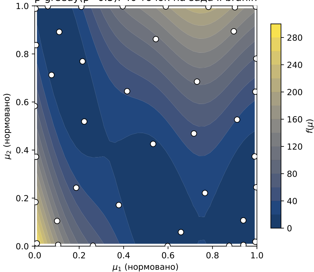
\beta -greedy( \beta=0.5 ): 40 точок на задачі branin
